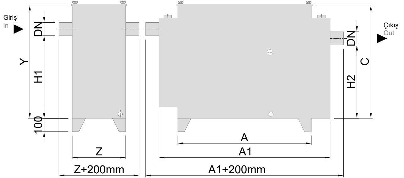
GÖRÜNÜŞ / ELEVATION
